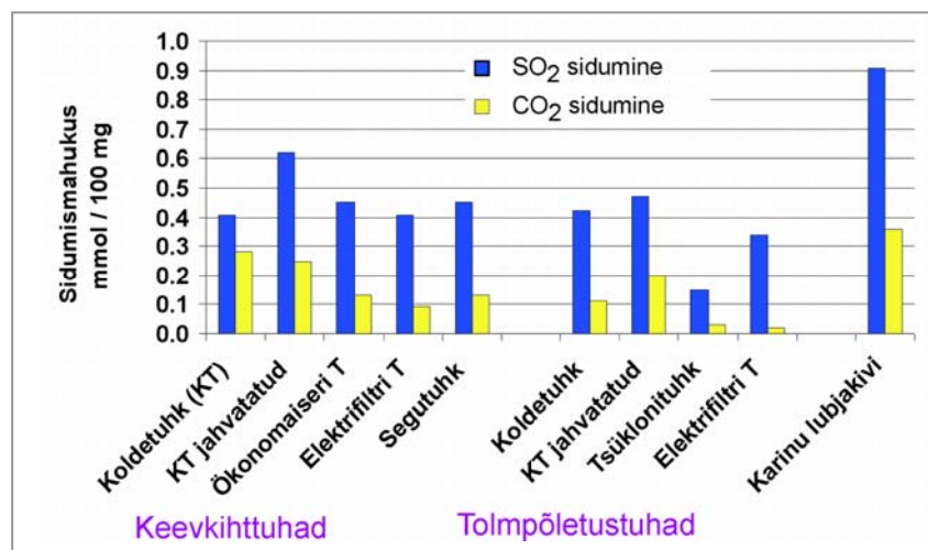
Joonis 4. Erinevate lubimaterjalide SO 2 ja CO 2 sidumismahukused (mmol gaasi 100 mg algproovi kohta) temperatuuril 700°C. p(SO 2 ) = 0,25 atm, p(CO 2 ) = 0,15 atm.
