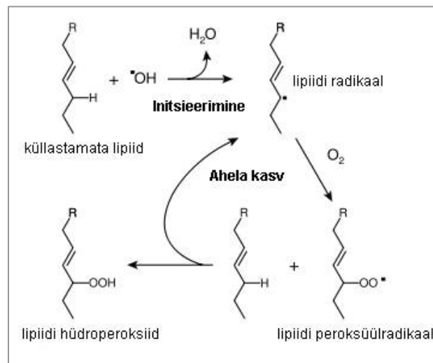
Joonis 2. Küllastamata lipiidi radikaalmehhanismiga oksüdeerimise algetapp.
