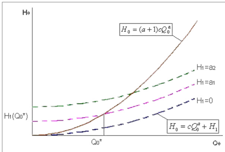
Joonis 10. Veevõrgu energiaetiliselt optimaalsed karakteristikud.
