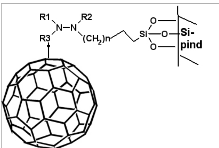
Joonis 2. Hüdrasiinosaani abil kovalentselt räni pinnale seotud fullereeni molekul. R1, R2, R3 on hüdrasiinosaani asendusrühmad, mille kaudu mõjutatakse süsteemi elektrilisi omadusi.
