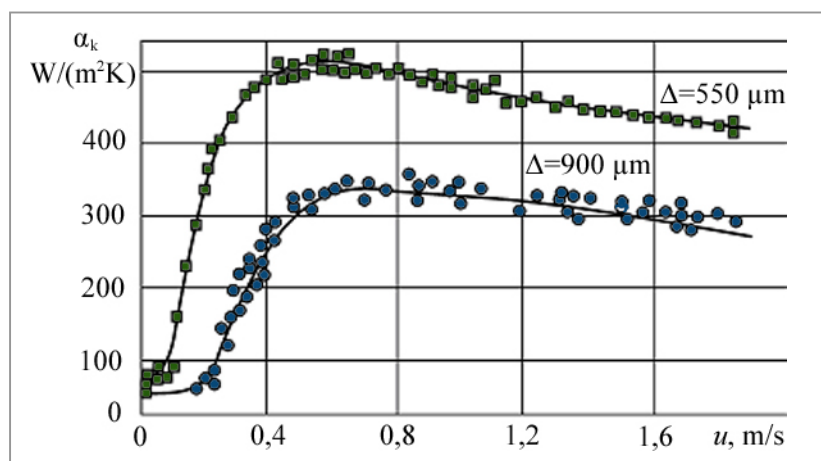
Joonis 3. Konvektiivsoojusülekande teguri sõltuvus gaasi kiirusest keevkihti asetatud silindrilisele kehale.
