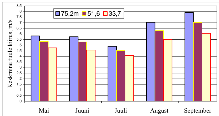
Joonis 2. Keskmised tuule kiirused Pakri tuulepargi asukohas kolmel kõrgusel 5 järjestikusel kuul (mai kuni september).
